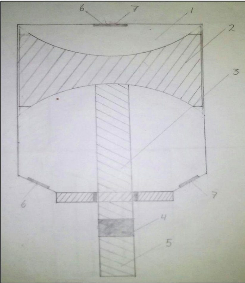
Fig. No- 2: Esquema del cilindro de un Motor de pistones alternativos
